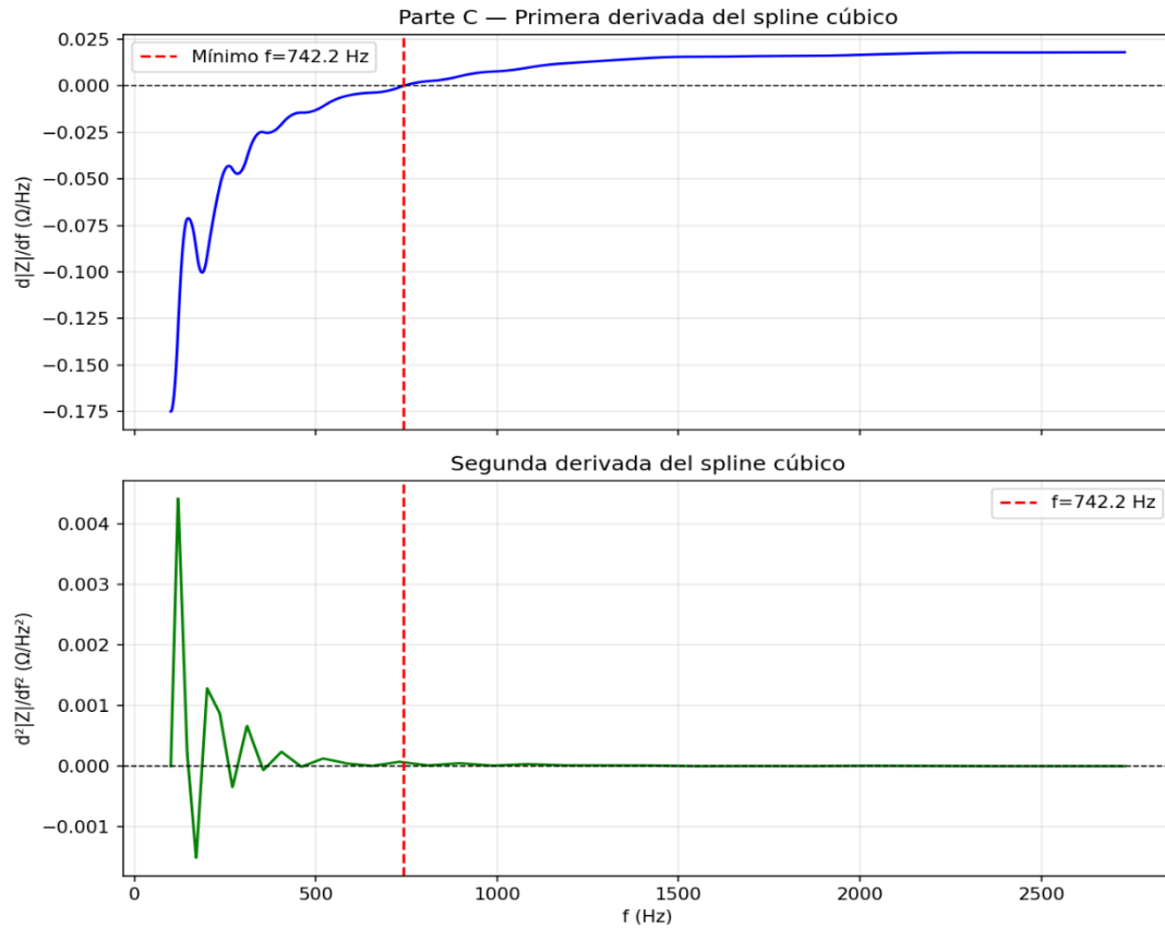
Figura 06: Primera y segunda derivada analítica del spline.
