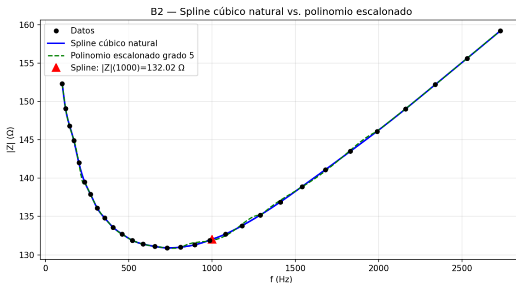
Figura 05: Spline cúbico natural vs. polinomio escalonado grado 5.
