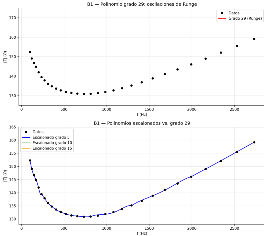
Figura04: Arriba: Runge en grado 29.
