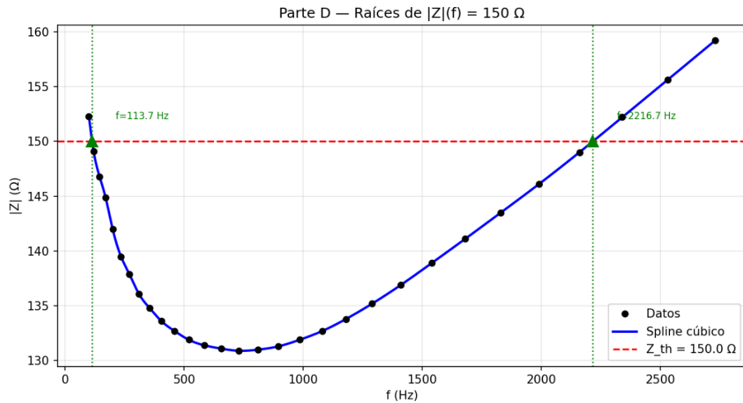
Figura 07: Spline y umbral Z_{th} = 150 \Omega . Raíces (triángulos verdes)
